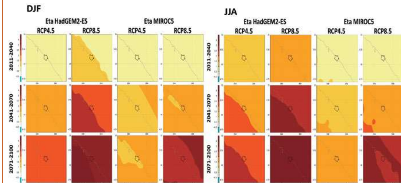
Figura 7.9 Projeções de temperatura do ar para DJF e JJA para a região de Fortaleza. Projeções para 2011-40, 2041-70 e 2071-2100 são relativas ao presente (1961-90), para os cenários RCP 4.5 e 8.5, derivados do downscaling dos modelos HadGEM2-ES e MIROC5 usando o modelo regional Eta.
