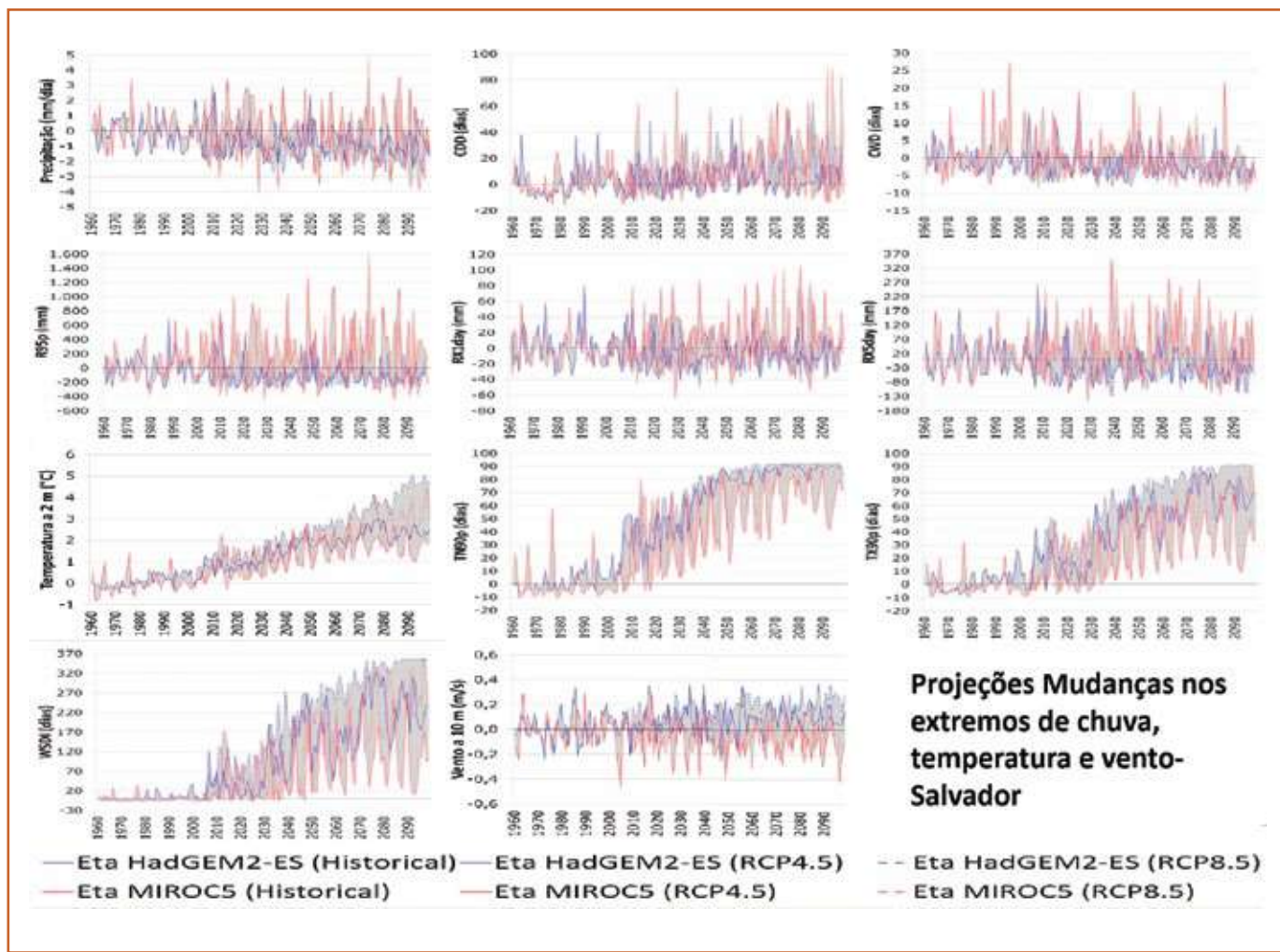
Figura 7.16 Tendência de anomalia da precipitação (mm/dia), dos índices extremos CDD (dias), CWD (dias), R95p (mm), RX1DAY (mm), RX5DAY (mm), da temperatura a 2 metros (°C), e os índices de extremos TN90p (dias), TX90p (dias), WSDI (dias), e vento a 10m (m/s) em Salvador, BA. Os valores médios da linha de base, período de 1961 a 1990, estão indicados na parte superior de cada gráfico. As anomalias foram calculadas a partir da diferença entre os valores anuais e o valor médio da linha de base. As anomalias das simulações do Eta-HadGEM2-ES (azul) e do Eta MIROC5 (vermelho) foram estimadas para os cenários futuros RCP4.5 (linha cheia) e RCP8.5 (linha tracejada). O intervalo de variação, entre os valores mínimos e máximos está hachurado em cinza.
