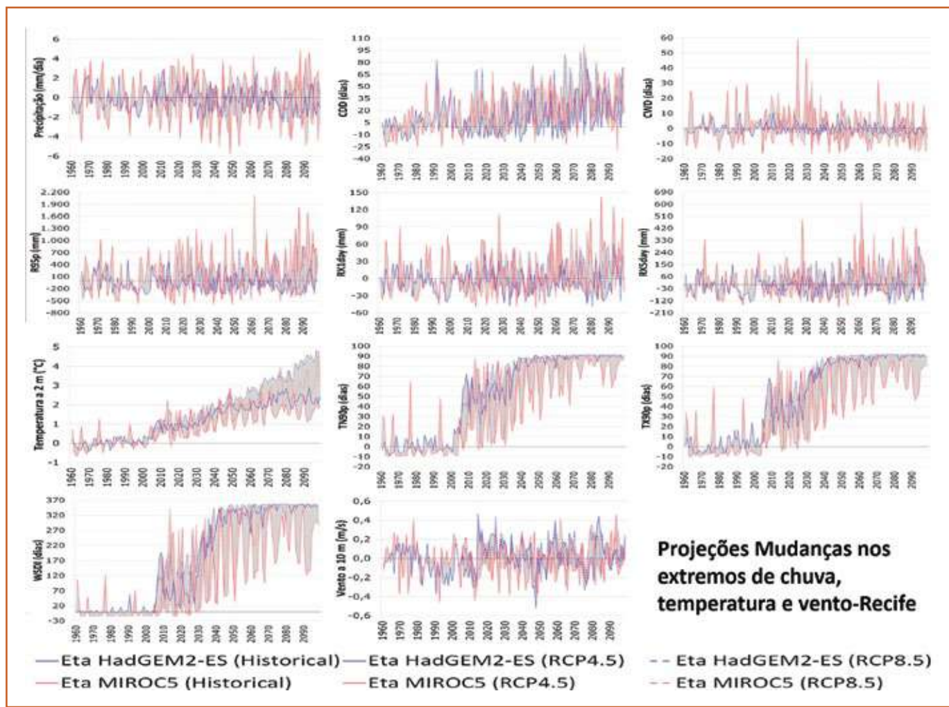
Figura 7.12 Tendência de anomalia da precipitação (mm/dia), dos índices extremos CDD (dias), CWD (dias), R95p (mm), RX1DAY (mm), RX5DAY (mm), da temperatura a 2 metros (°C), e os índices de extremos TN90p (dias), TX90p (dias), WSDI (dias), e vento a 10m (m/s) no Recife, PE. Os valores médios da baseline, período de 1961 a 1990, estão indicados na parte superior de cada gráfico. As anomalias foram calculadas a partir da diferença entre os valores anuais e o valor médio da baseline. As anomalias das simulações do Eta-HadGEM2-ES (azul) e do Eta-MIROC5 (vermelho) foram estimadas para os cenários futuros RCP4.5 (linha cheia) e RCP8.5 (linha tracejada). O intervalo de variação, entre os valores mínimos e máximos está hachurado em cinza.
