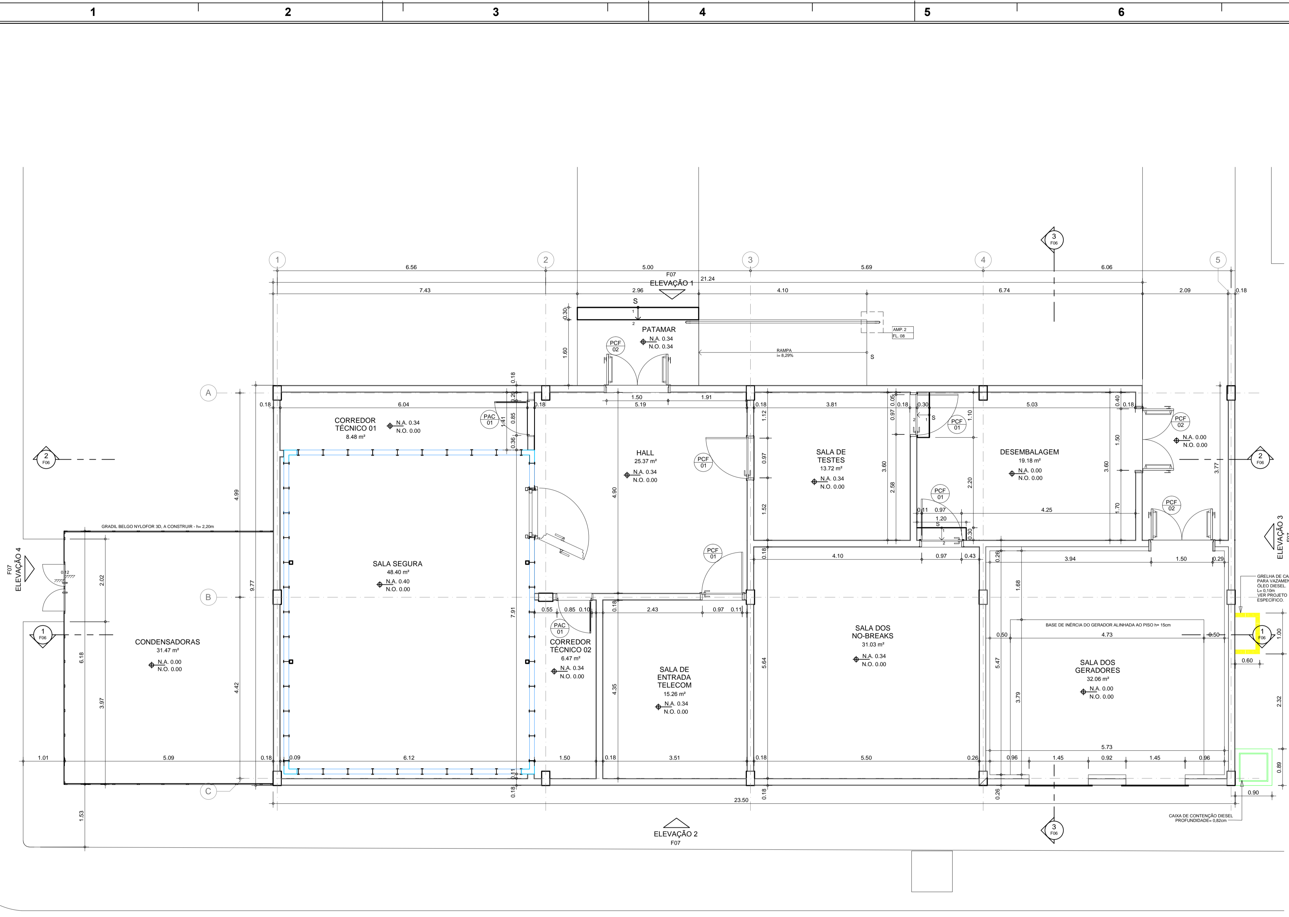
1 PLANTA DE CONSTRUÇÃO - PAVIMENTO TÉRREO 1:50
