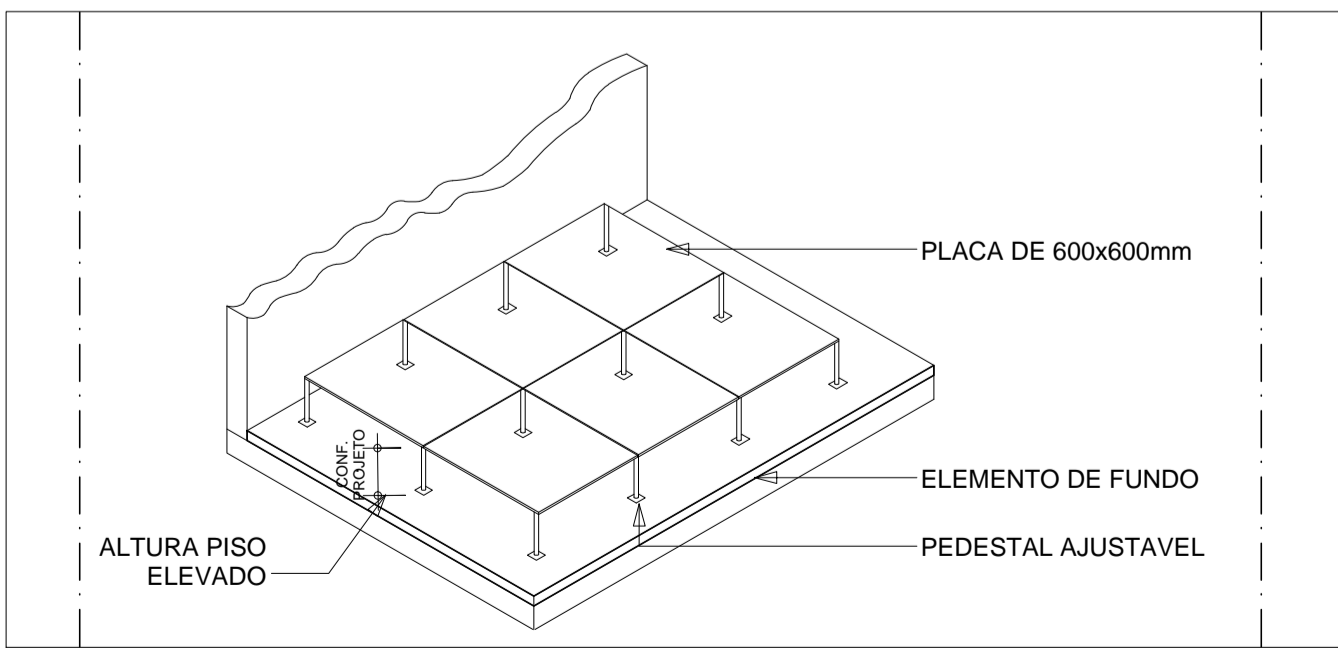
1 DET. PISO ELEVADO EM PERSPECTIVA 1:15
