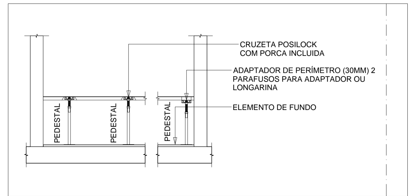
2 DET. PISO ELEVADO EM CORTE 1:20
