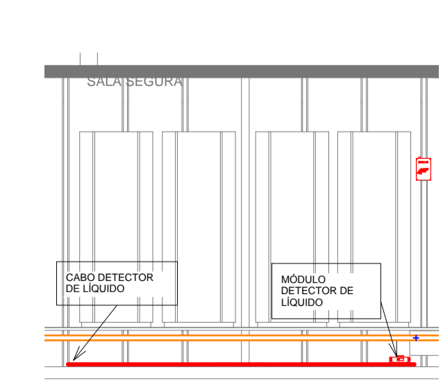
4 DETECTOR DE LÍQUIDO 1:50
