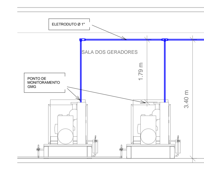
6 DETALHES DE INSTALAÇÃO PONTOS GMG 1:50
