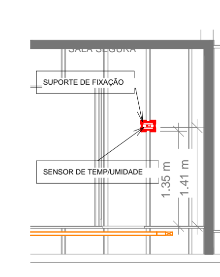
5 SENSOR DE TEMPERATURA SALA SEGURA 1:50
